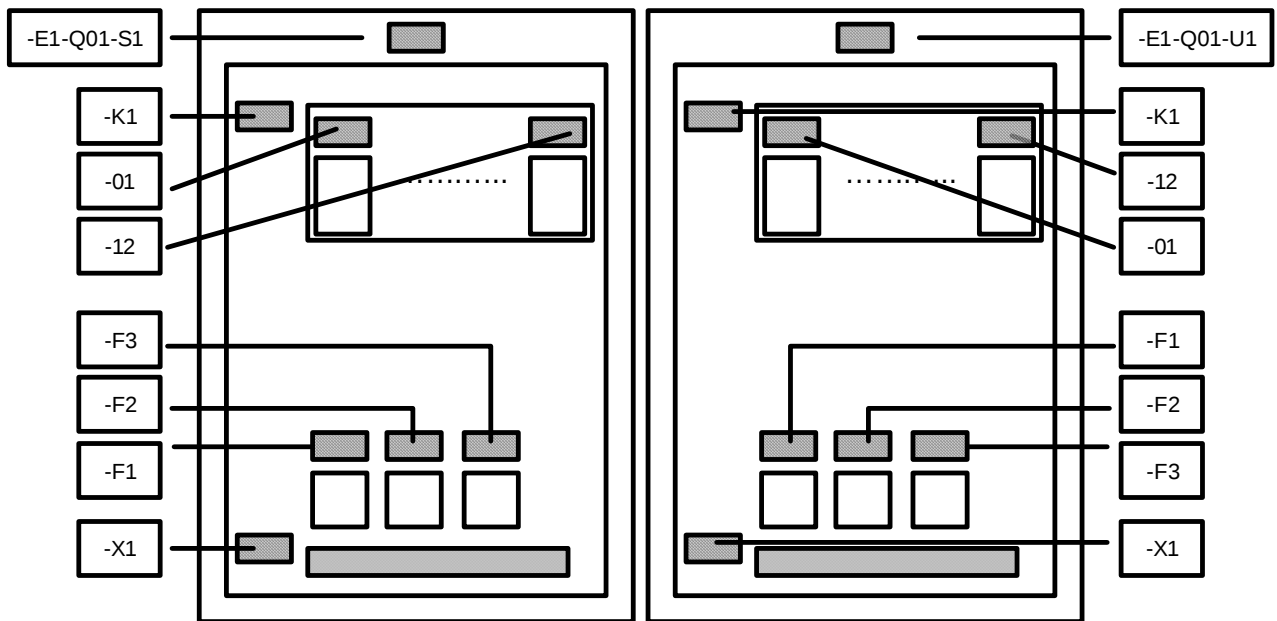
Abbildung 25 - Aufgeteilte Darstellung von Referenzkennzeichen
