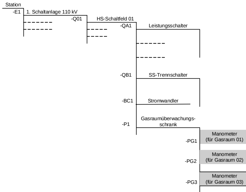
Abbildung 23 – Kontaktmanometer in feldbezogenem Gasüberwachungsschrank
