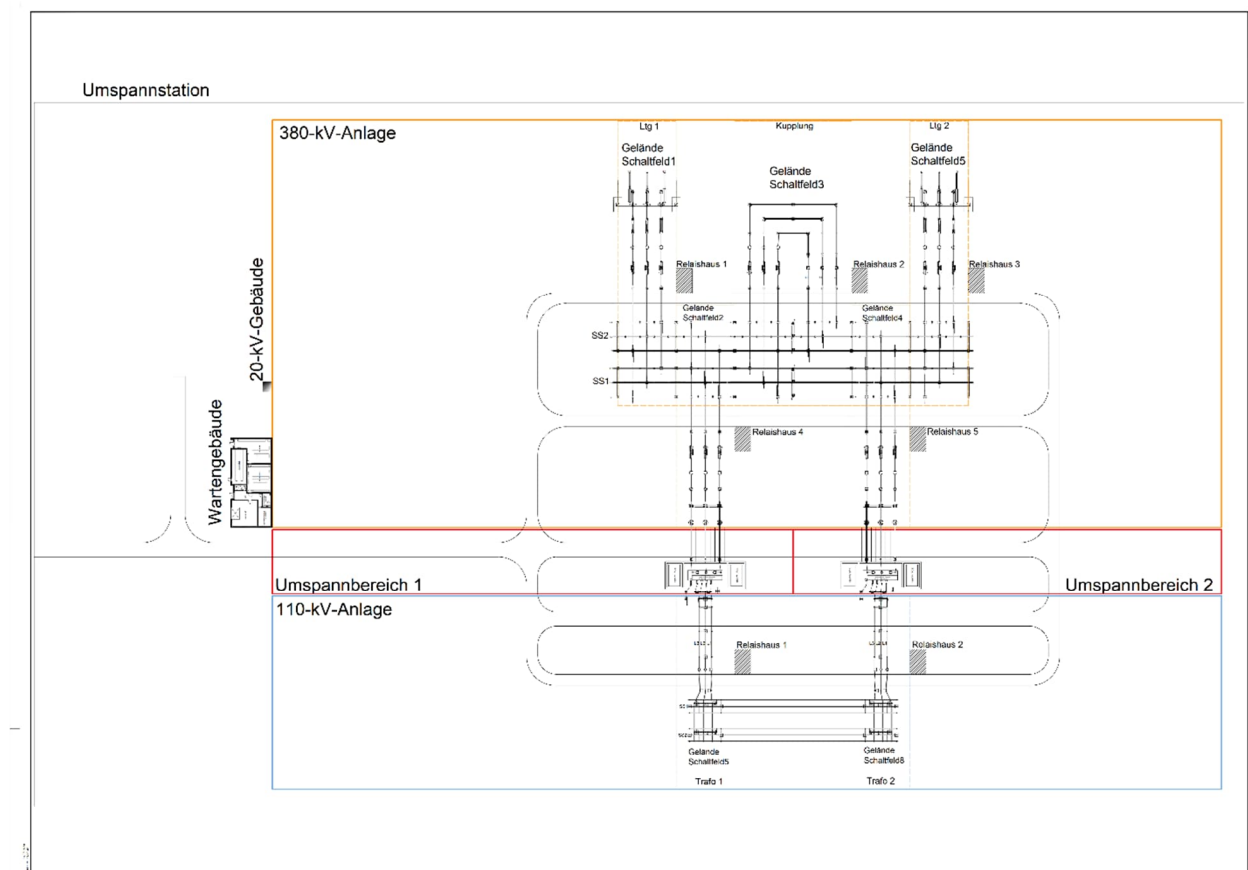
Abbildung 3 – Beispiel einer Umspannstation – Grundriss
