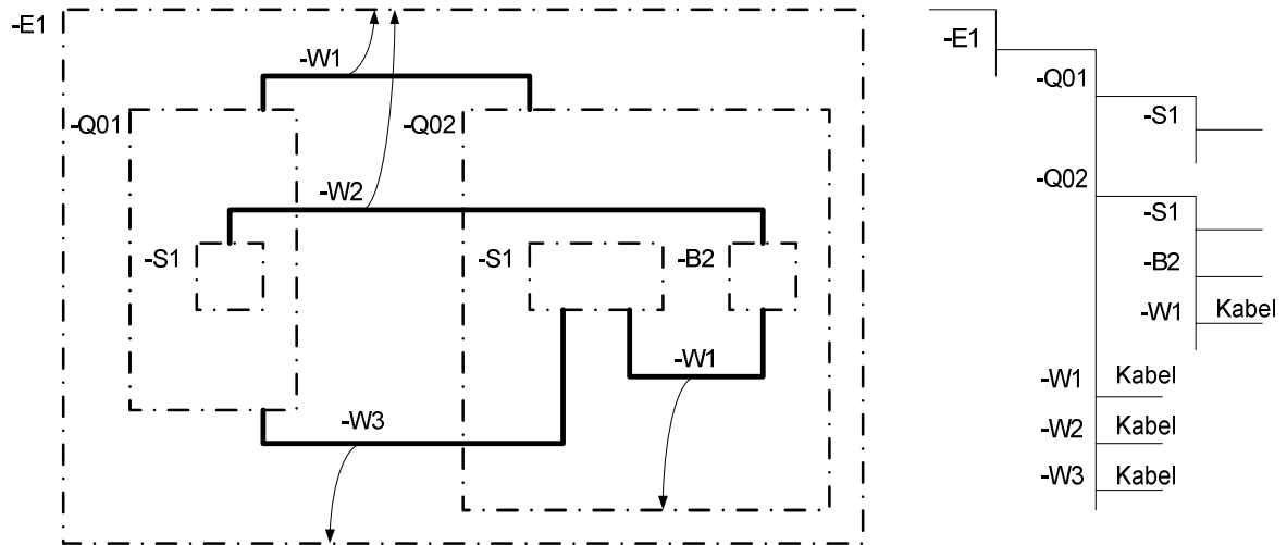
Abbildung 11 - Prinzip der Kabelkennzeichnung
