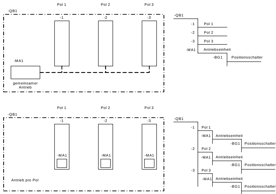
Abbildung 17 – Beispiele für die Kennzeichnung von Trennschaltern in verschiedenen Bauformen
