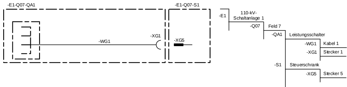
Abbildung 15 – Kennzeichnung von Kabeln mit Steckern
