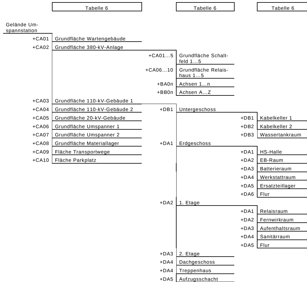
Abbildung 9 – Beispiel für ortsbezogene Struktur mit Referenzkennzeichen
