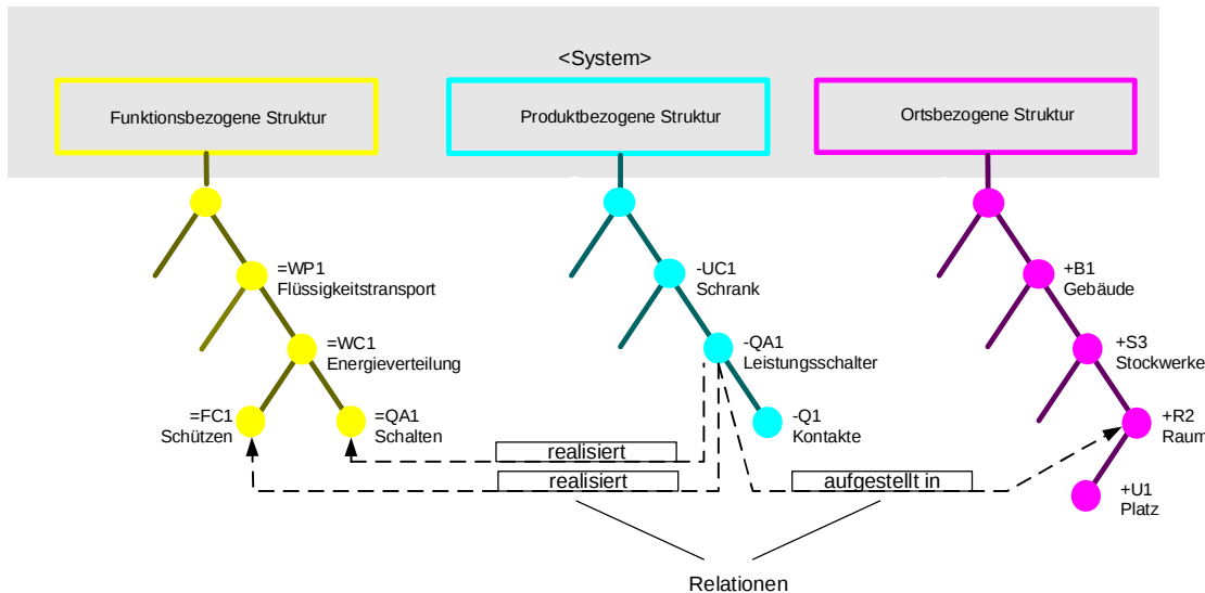
Abbildung 10 – Referenzkennzeichensatz dokumentiert Beziehungen zwischen Objekten
