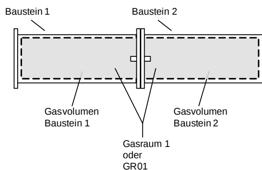
Abbildung 21 – Gasraum, bausteinübergreifend
