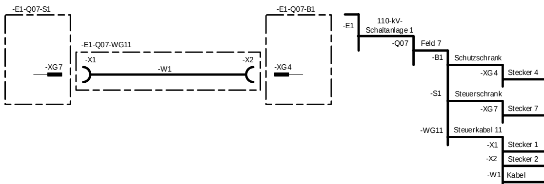
Abbildung 13 – Kennzeichnung von Kabeln mit Steckern
