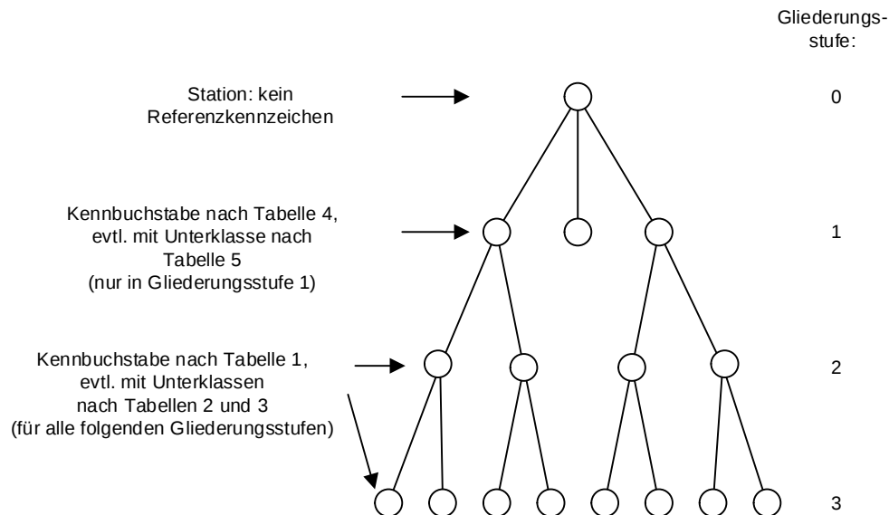
Abbildung 6 – Zuordnung der Klassifizierungstabellen zu den Gliederungsstufen in den Anlagenstrukturen
