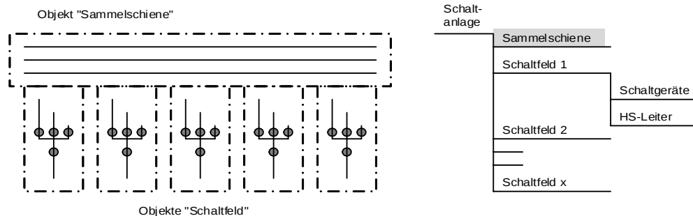
Beispiel "Freiluftschaltanlage"
