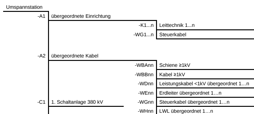
Abbildung 12 – Beispiel für Kabel auf Stationsebene in der Produktstruktur
