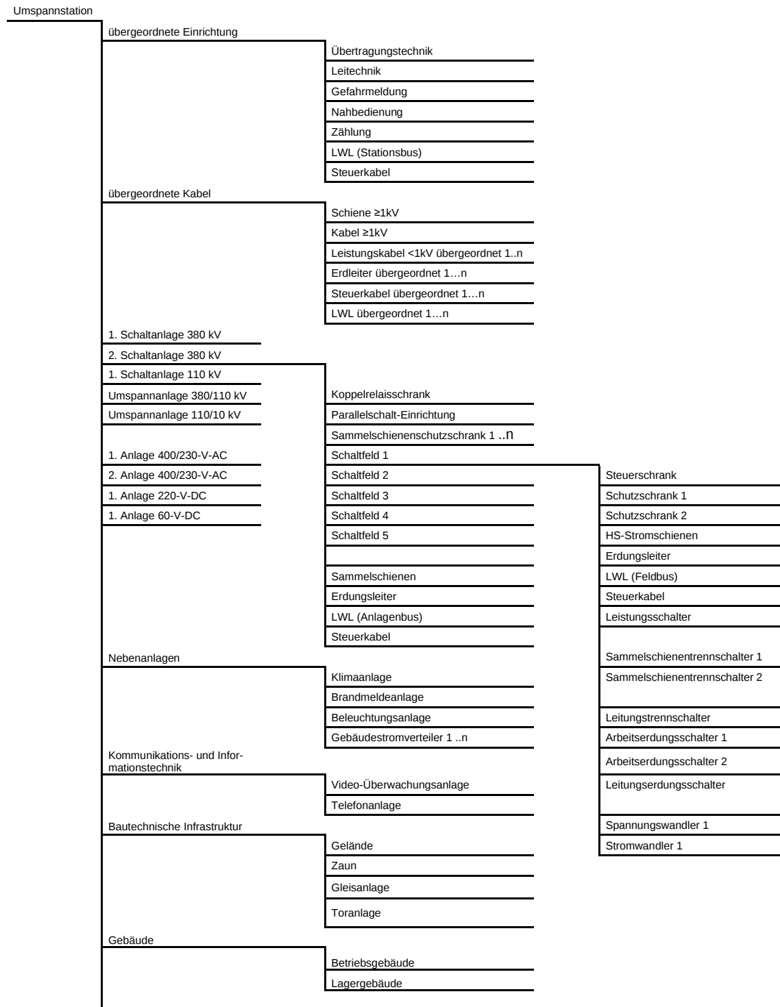
Abbildung 2 – Beispiel einer produktbezogenen Struktur
