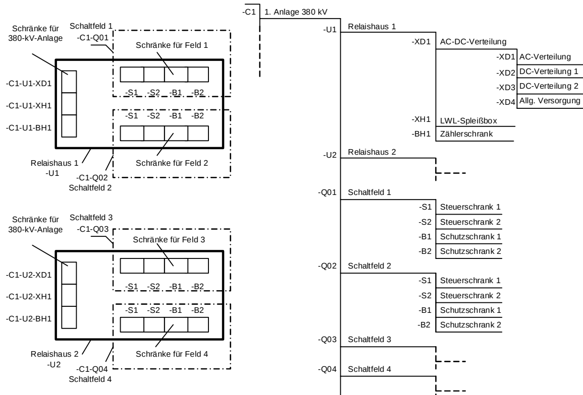
Abbildung 16 – Kennzeichnung von Objekten in Relais Häusern
