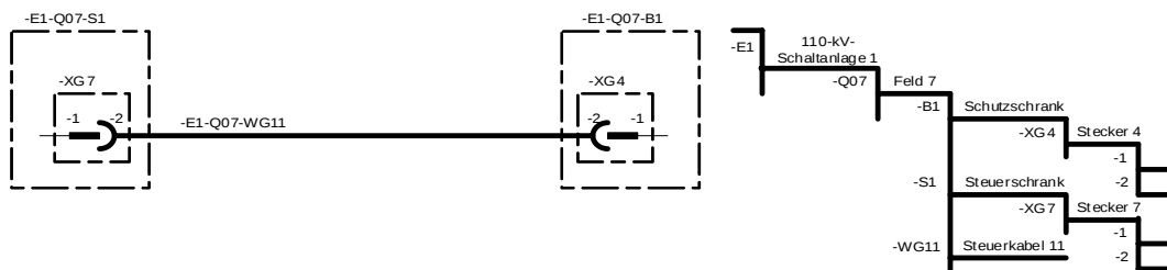
Abbildung 14 – Kennzeichnung von Kabeln mit Steckern
